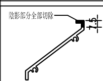
②號百葉加工圖
