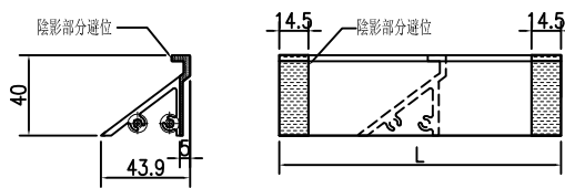
③號百葉加工圖
