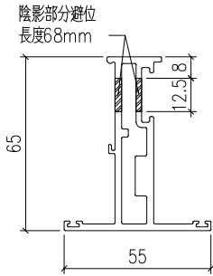
剖面B-B
