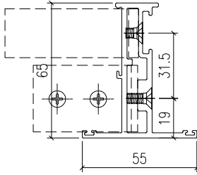
剖面A-A
