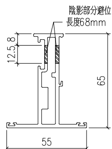
剖圖B-B
