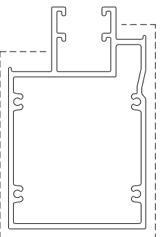
模號: X86061 名稱: 側窗中橫 合金狀態: 6063-T6 重量: 6.483 KG/M V.F.: 0.4265 m 2 /m
