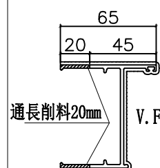
削料示意圖
