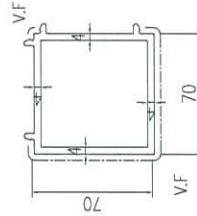
模號: X86009 名稱: 90°轉角通 合金狀態: 6063-T6 重量: 3.055KG/M V.F.: 150mm
