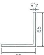
模號: X86021 名稱: 70窗斜角 合金狀態: 6061-T6 重量: 1.530KG/M V.F.: 0mm
