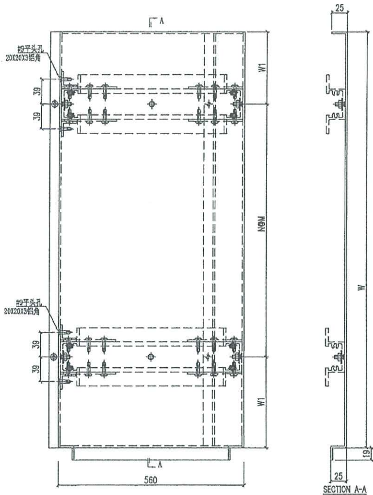
SECTION A-A
