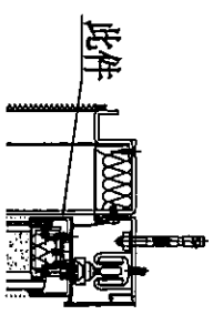
鋁折件修改安裝示意圖
