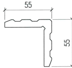
模號: X86466 名稱: L角碼 合金狀態: 6063-T6 重量: 2.207KG/M V.F.: 0 mm
