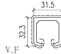
模號: X86467 名稱: 導軌 合金狀態: 6063-T6 重量: 0.892KG/M V.F.: 118.94mm
