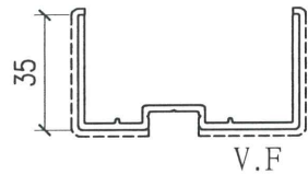
模號: X86494 名稱: 外框料 合金狀態: 6063-T6 重量: 0.784KG/M V.F.: 217 mm
