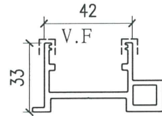
模號: X86465 名稱: 內框料 合金狀態: 6063-T6 重量: 1.124KG/M V.F.: 35 mm 噴塗有問題待香港定
