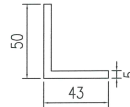
模號: JMA0553 名稱: 50X43X5鋁角 合金狀態: 6063-T5 重量: 1.287KG/M V.F.: 0 mm
