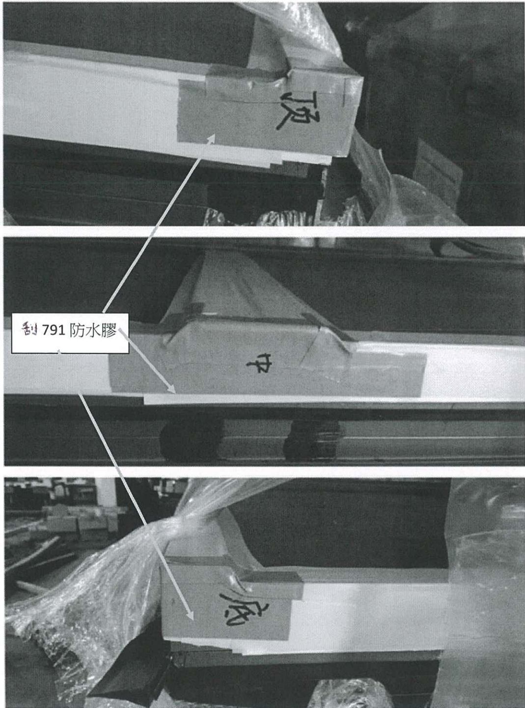
刮 791 防水膠在膠紙面以加強幕牆單元膠紙的保護
