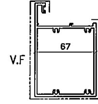
模號: X86480 名稱: 梗勾企 合金狀態: 6063-T6 重量: 2.399KG/M V.F.: 260.64 mm
