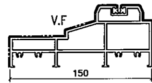
模號: X86492 名稱: 雙趟框底橫 合金狀態: 6063-T6 重量: 3.869KG/M V.F.: 389.08 mm
