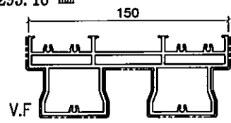
模號: X86491 名稱: 雙趟框頂橫 合金狀態: 6063-T6 重量: 4.460KG/M V.F.: 403.68 mm
