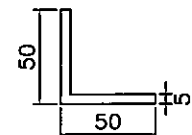
模號: JM1001 名稱: 50X50X5鋁角 合金狀態: 6063-T5 重量: 1.390KG/M V.F.: 0 mm
