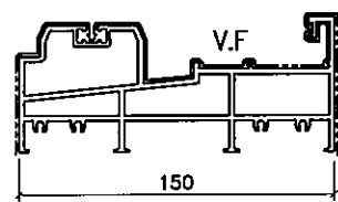
模號: X86490 名稱: 單趟框底橫 合金狀態: 6063-T6 重量: 4.289KG/M V.F.: 460.44 mm
