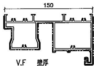
模號: X86489 名稱: 單趟框頂橫 合金狀態: 6063-T6 重量: 4.071KG/M V.F.: 480.35 mm
