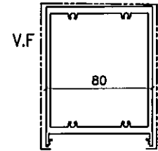
模號: X86484 名稱: 玉拉手料 合金狀態: 6063-T6 重量: 3.994KG/M V.F.: 293.16 mm
