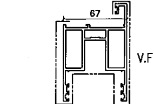
模號: X86476 名稱: 玉玻線 合金狀態: 6063-T5 重量: 0.251KG/M V.F.: 90.64 mm
