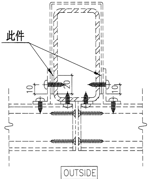
安裝示意圖
