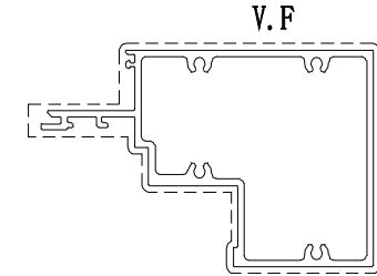
模號: AT04 名稱: 生窗中橫 合金狀態: 6063-T6 重量: 4.54 KG/M V.F.: 0.566 m 2 /m
