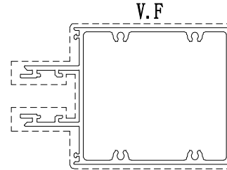
模號: AT03 名稱: 梗窗中橫 合金狀態: 6063-T6 重量: 4.96 KG/M V.F.: 0.707 m 2 /m
