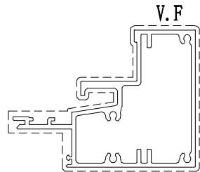
模號: AT05 名稱: 生窗中橫 合金狀態: 6063-T6 重量: 4.66 KG/M V.F.: 0.584 m 2 /m
