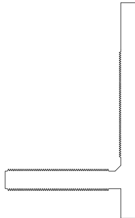
模號: ABO1 名稱: 牆邊鋁碼 合金狀態: 6061-T6 重量: 16.25 KG/M V.F.: 0 m 2 /m
