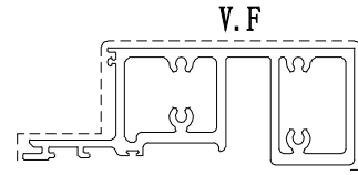
模號: AT02 名稱: 底橫料 合金狀態: 6063-T6 重量: 5.653 KG/M V.F.: 0.284 m 2 /m
