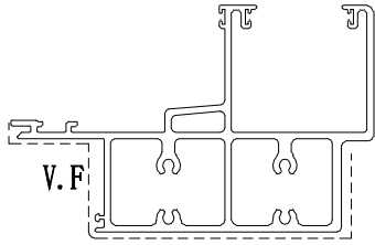
模號: AT01 名稱: 頂橫料 合金狀態: 6063-T6 重量: 6.03 KG/M V.F.: 0.272 m 2 /m
