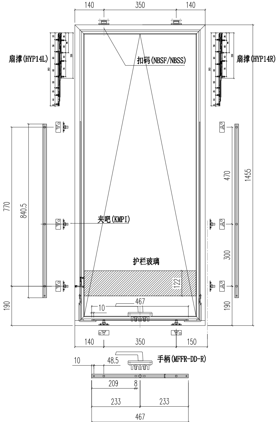
T, H 窗按单元中至中650尺寸放样
