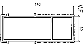
模號: IT-06 名稱: (140X50) 中企夾通 合金狀態: 6063-T5 重量: 5.728KG/M V.F.: 272mm
