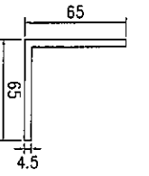
模號: X86021 名稱: 70寬斜角 合金狀態: 6061-T6 重量: 1.530KG/M V.F.: 0mm
