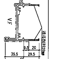
模號: X86014 名稱: 70生頂機 合金狀態: 6063-T6 重量: 1.347KG/M V.F.: 220.19mm
