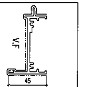
模號: X86006 名稱: 70邊來企 合金狀態: 6063-T6 重量: 0.838KG/M V.F.: 188.41mm
