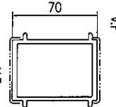
模號: X86108 名稱: 中企夾通(70mm) 合金狀態: 6063-T6 重量: 2.285KG/M V.F.: 168.21mm
