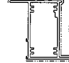
模號: X86015 名稱: 70上生下機中機 合金狀態: 6063-T6 重量: 1.838KG/M V.F.: 233.49mm
