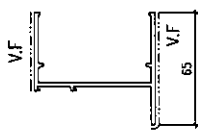
模號: X86005 名稱: 70側邊企 合金狀態: 6063-T6 重量: 1.151KG/M V.F.: 228.15mm
