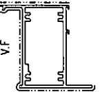
模號: X86015 名稱: 70上生下橫中橫 合金狀態: 6063-T6 重量: 1.838KG/M V.F.: 233.49mm
