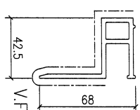
模號: X86498 名稱: 竖向玻璃框 合金狀態: 6063-T6 重量: 1.331 KG/M V.F.: 162.9 mm
