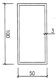
模號: JMF0032B30 名稱: 100x50x3mm铝通 合金狀態: 6063-T6 重量: 2.528 KG/M V.F.: -
