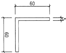
模號: X86514 名稱: 码件垫片 合金狀態: 6061-T6 重量: 1.789 KG/M V.F.: -
