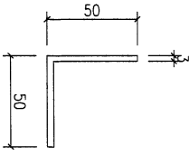
模號: JM1001 名稱: 50x50x3mm铝角 合金狀態: 6063-T6 重量: 0.852 KG/M V.F.: -
