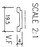
模號: X86508 名稱: 开窗连杆 合金狀態: 6063-T6 重量: 0.129 KG/M V.F.: 29.29mm
