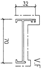
模號: X85951 名稱: 百叶副框 合金狀態: 6063-T6 重量: 0.85 KG/M V.F.: 178.36mm
