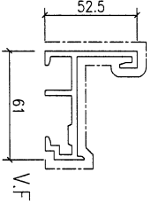
模號: X86505 名稱: 开窗竖向内框 合金狀態: 6063-T6 重量: 1.442 KG/M V.F.: 208.97mm
