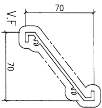
模號: X85958 名稱: 百叶片 合金狀態: 6063-T6 重量: 1.04 KG/M V.F.: 272.52mm
