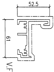
模號: X86509 名稱: 开窗横向内框 合金狀態: 6063-T6 重量: 1.503 KG/M V.F.: 225.21mm
