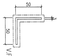
模號: JM1001 名稱: 50x50x3mm铝角 合金狀態: 6063-T6 重量: 0.852 KG/M V.F.: 200mm
