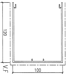
模號: X86495 名稱: 包鋼型材 合金狀態: 6063-T6 重量: 2.353 KG/M V.F.: 442.07mm
