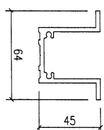
模號: X86271 名稱: 铝板加力筋 合金狀態: 6063-T6 重量: 1.727 KG/M V.F.: - mm
