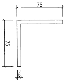
模號: JM1079 名稱: 75x75x6mm铝角 合金狀態: 6063-T6 重量: 2.539 KG/M V.F.: -
