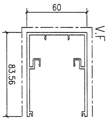
模號: X86449 名稱: 包鋼型材 合金狀態: 6063-T6 重量: 1.772 KG/M V.F.: 354.28mm
