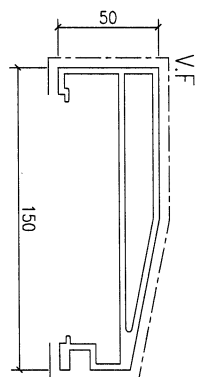
模號: X86452 名稱: 扶手面管 合金狀態: 6063-T6 重量: 3.46 KG/M V.F.: 315.49mm
