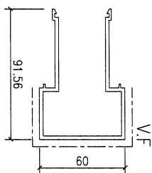
模號: X86450 名稱: 包鋼型材 合金狀態: 6063-T6 重量: 1.781 KG/M V.F.: 327.06mm
