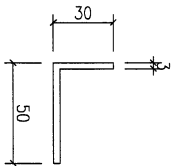
模號: JM1030 名稱: 50x30x3mm鋁角 合金狀態: 6063-T6 重量: 0.676 KG/M V.F.: - mm
