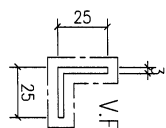
模號: JM1015 名稱: 25x25x3mm鋁角 合金狀態: 6063-T6 重量: 0.413 KG/M V.F.: 100 mm
