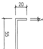
模號: JM1003 名稱: 55x20x3mm鋁角 合金狀態: 6063-T6 重量: 0.632 KG/M V.F.: - mm
