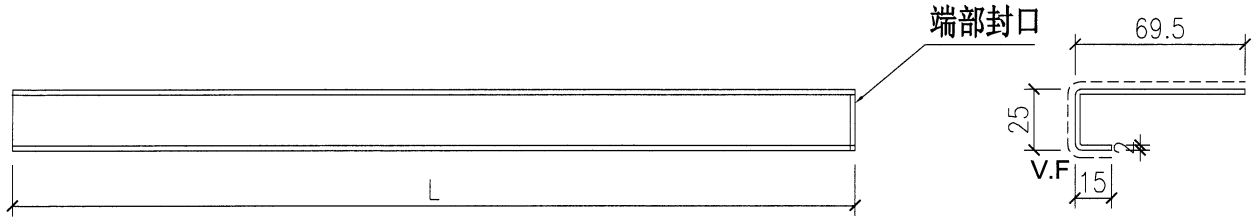
封口示意图
