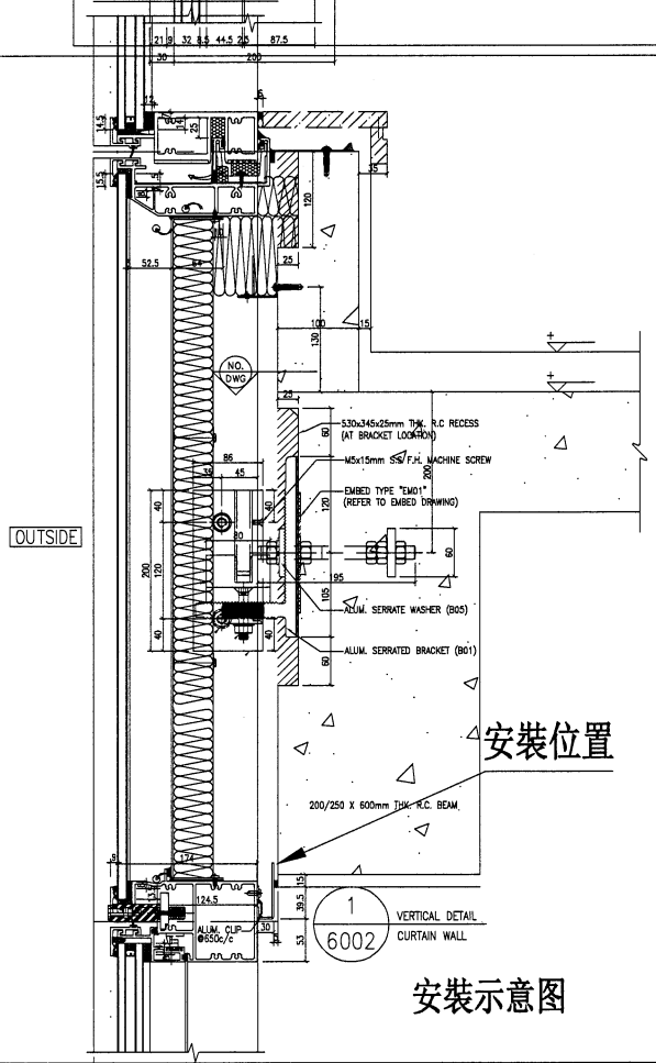
安裝示意图
