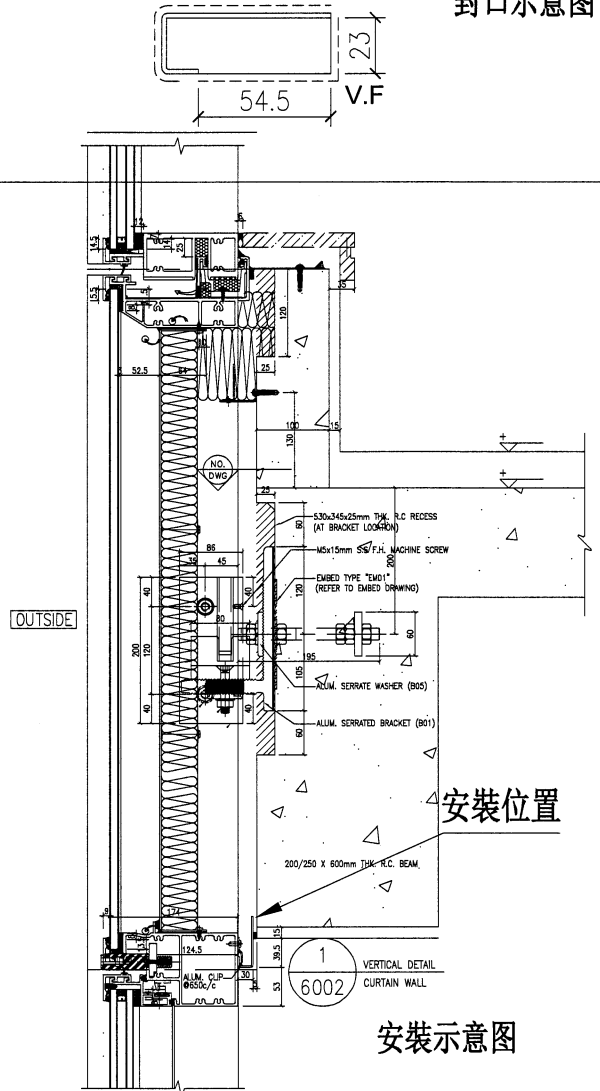
封口示意图
