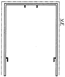
模號: X86401 名稱: 裝飾條外蓋 合金狀態: 6063-T6 重量: 2.583KG/M V.F.: 478.1 mm
