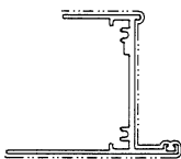
模號: X86947 名稱: 生底橫 合金狀態: 6063-T6 重量: 1.327KG/M V.F.: 237.08 mm
