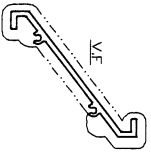
模號: X85958 名稱: 70百葉片 合金狀態: 6063-T6 重量: 1.068KG/M V.F.: 272 mm
