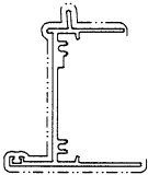
模號: X86946 名稱: 生頂橫 合金狀態: 6063-T6 重量: 1.233KG/M V.F.: 234.97 mm
