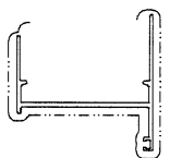
模號: X86948 名稱: 生底企 合金狀態: 6063-T6 重量: 1.057KG/M V.F.: 217.9 mm
