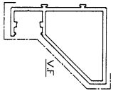
模號: X86415 名稱: 裝飾條 合金狀態: 6063-T6 重量: 1.686KG/M V.F.: 163.5 mm
