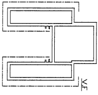
模號: X86413 名稱: 裝飾條 合金狀態: 6063-T6 重量: 4.062KG/M V.F.: 310.3 mm
