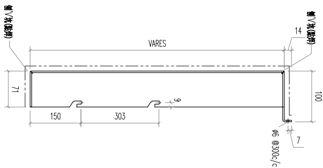
SECTION A2-A2
