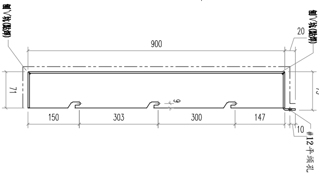
SECTION A2-A2
