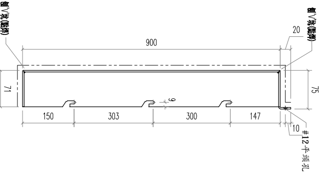
SECTION A2-A2
