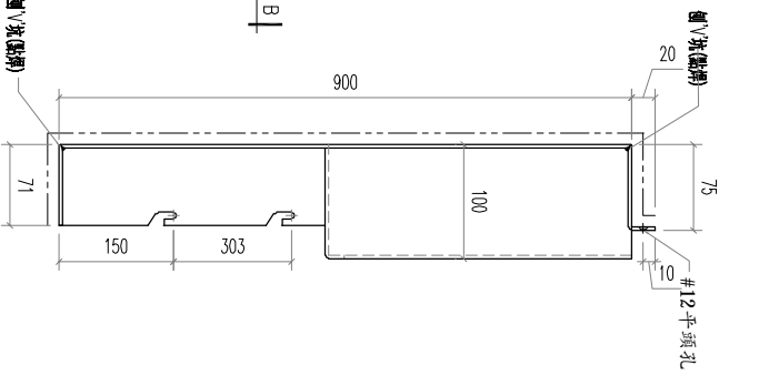
SECTION A2-A2
