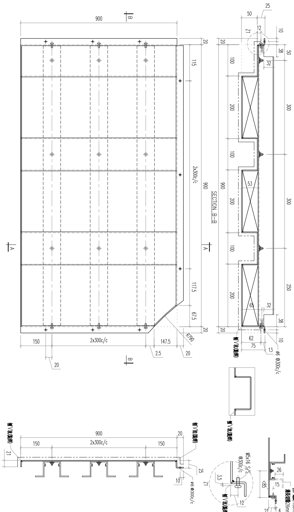
SECTION A-A
