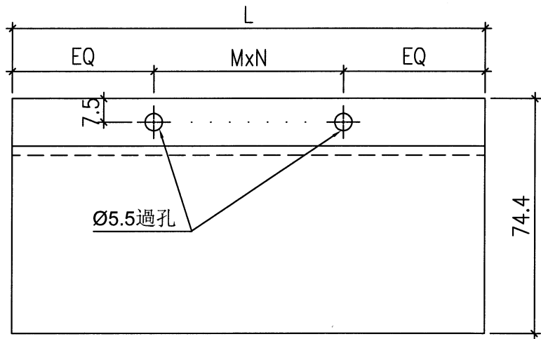
安裝示意圖
