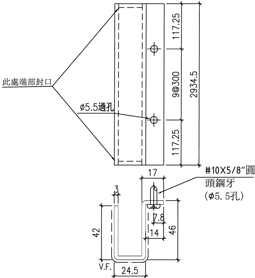
安裝示意圖
