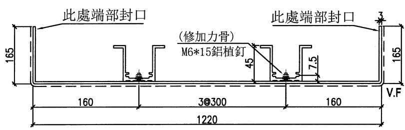
剖面B-B
