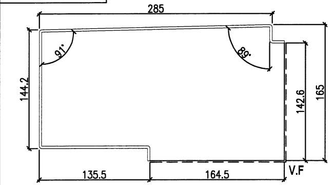
端部封口示意圖
