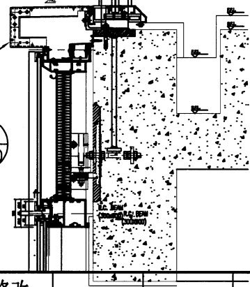
安裝示意圖
