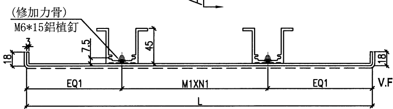
剖面B-B
