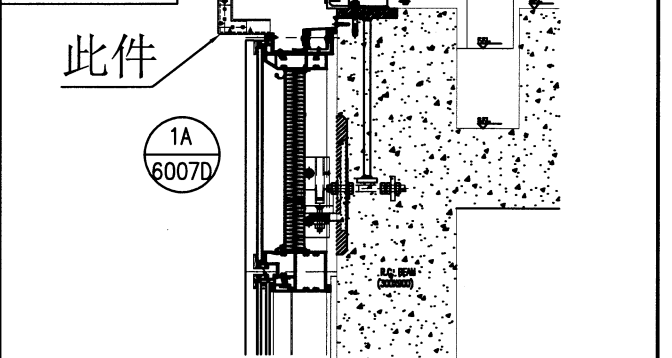
安裝示意圖
