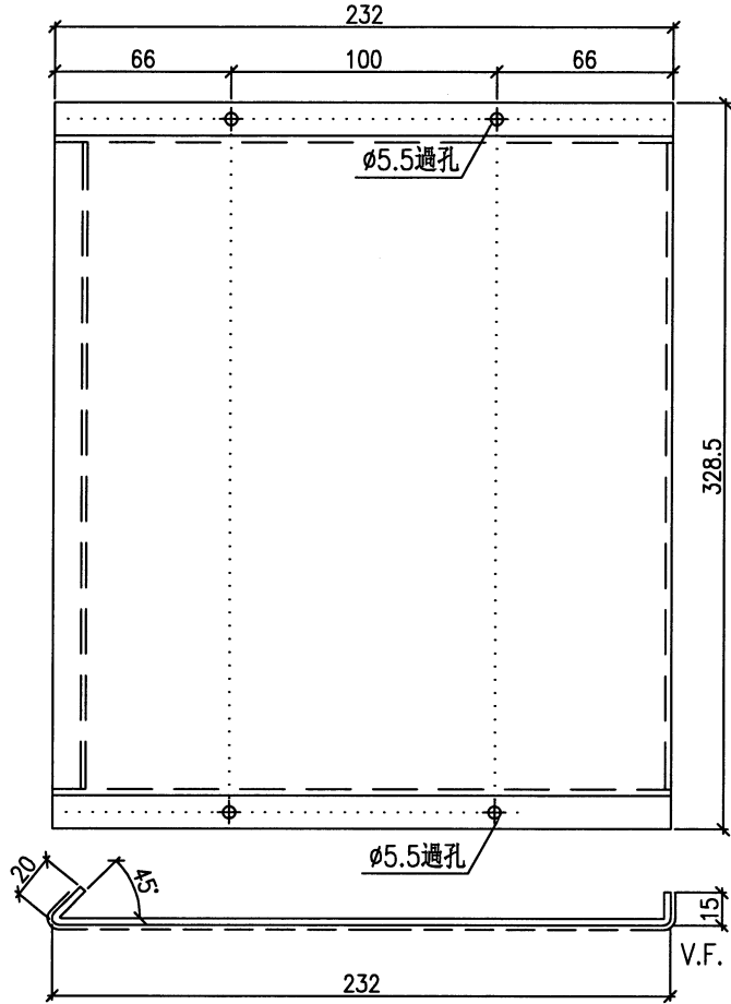
安裝示意圖
