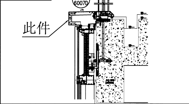
安裝示意圖
