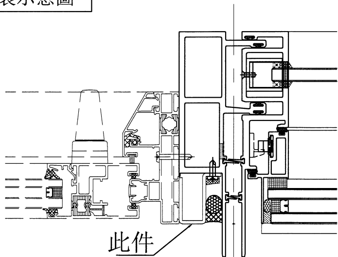
安裝示意圖
