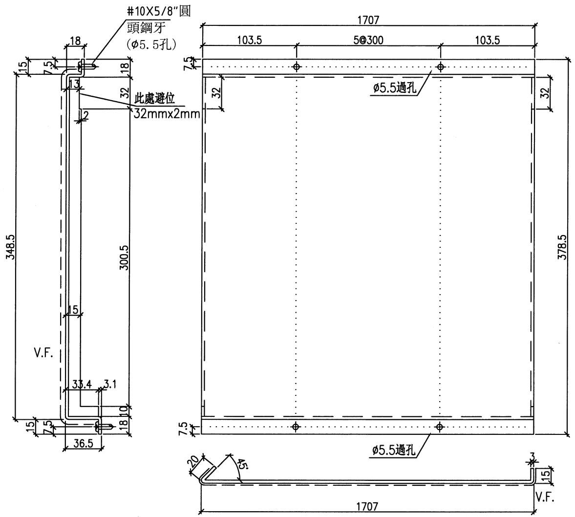
安裝示意圖
