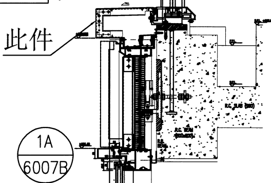
安裝示意圖
