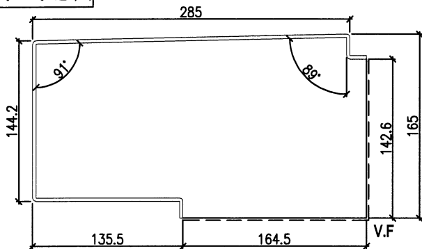
端部封口示意圖
