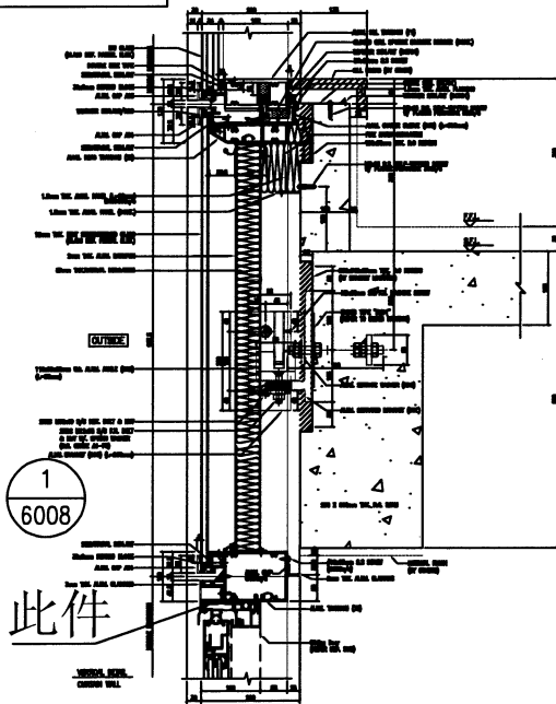
安裝示意圖
