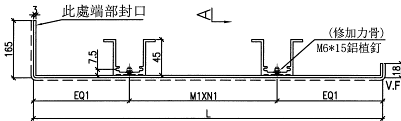
剖面B-B
