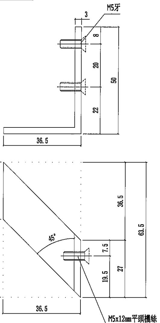
安裝示意圖
