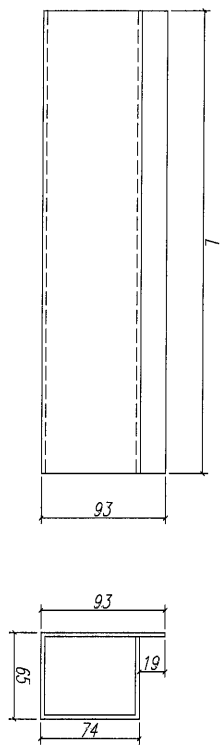
鋁折件13/14
