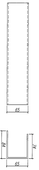
鋁折件1
