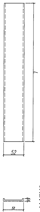
鋁折件15/16
