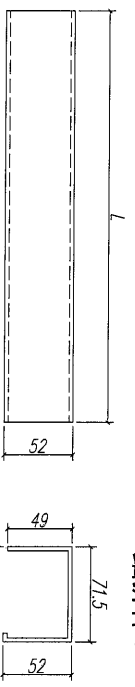
鋁折件4
