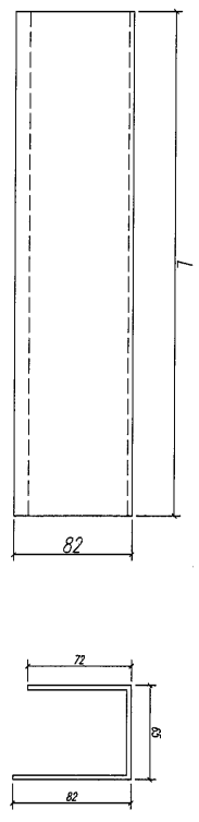
鋁折件15/16
