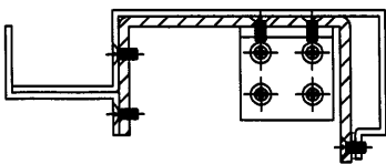
安裝示意
