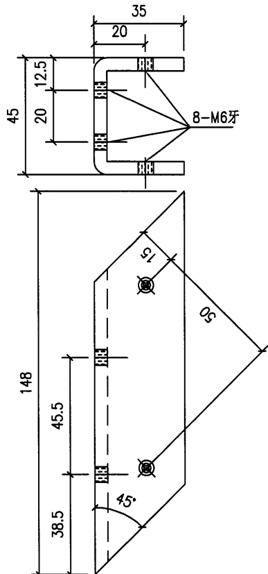
J853-M2-1 数量:20个
