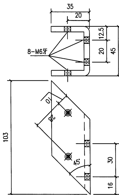
J853-M2-3
