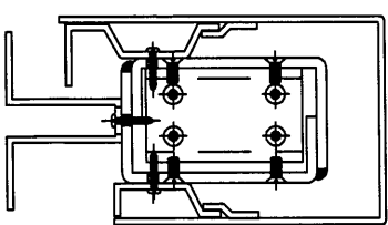
安裝示意
