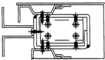
安裝示意
