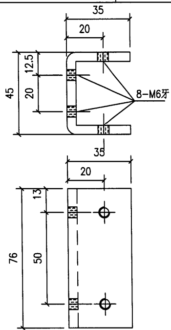
J853-M1-3 數量:50个
