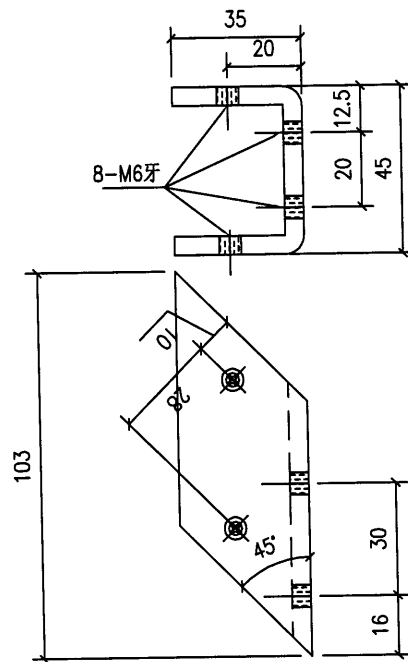
J853-M2-3 数量:20个
