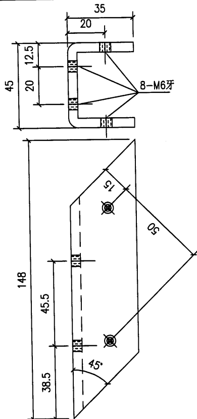
J853-M2-1 数量:20个
