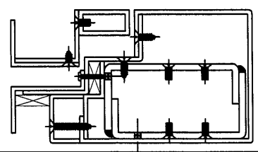
安裝示意
