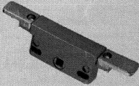
2035-A双向 行程:19mm
