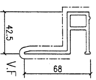
模號: X86498 名稱: 豎向玻璃框 合金狀態: 6063-T6 重量: 1.331 KG/M V.F.: 162.9mm
