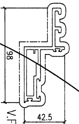
模號: X86507 名稱: 开窗橫向外扇 合金狀態: 6063-T6 重量: 1.849 KG/M V.F.: 353.78mm
