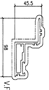
模號: X86506 名稱: 开窗竖向外扇 合金狀態: 6063-T6 重量: 1.722 KG/M V.F.: 332.86mm
