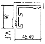
模號: X86500 名稱: 开窗玻璃扣条 合金狀態: 6063-T6 重量: 0.884 KG/M V.F.: 131.67mm
