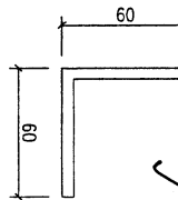
模號: JM1069 名稱: 60x60x5mm鋁角 合金狀態: 6061-T6 重量: 1.883 KG/M V.F.: -
