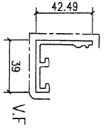
模號: X86499 名稱: 玻璃扣条 合金狀態: 6063-T6 重量: 0.844 KG/M V.F.: 122.52mm
