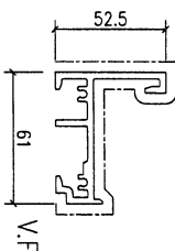
模號: X86509 名稱: 开窗橫向内框 合金狀態: 6063-T6 重量: 1.503 KG/M V.F.: 225.21mm
