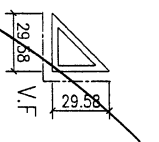
模號: X86510 名稱: 轉角墊高料 合金狀態: 6063-T6 重量: 0.691 KG/M V.F.: 60.56
