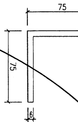
模號: JM1079 名稱: 75x75x6mm鋁角 合金狀態: 6063-T6 重量: 2.539 KG/M V.F.: -
