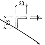
模號: JM1012A 名稱: 20x20x3mm鋁角 合金狀態: 6063-T6 重量: 0.325 KG/M V.F.: -
