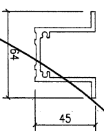
模號: X86271 名稱: 铝板加力筋 合金狀態: 6063-T6 重量: 1.727 KG/M V.F.: -
