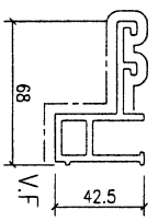
模號: X86501 名稱: 橫向玻璃框 合金狀態: 6063-T6 重量: 1.497 KG/M V.F.: 184.49mm
