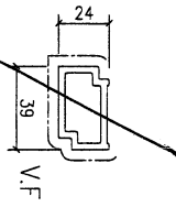
模號: X86512 名稱: 豎向墊高料 合金狀態: 6063-T6 重量: 0.926 KG/M V.F.: 81.93
