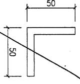
模號: X86515 名稱: 50x50x7.2mm鋁角 合金狀態: 6063-T6 重量: 1.811 KG/M V.F.: -
