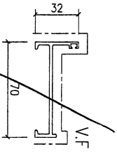
模號: X85951 名稱: 百叶副框 合金狀態: 6063-T6 重量: 0.85 KG/M V.F.: 178.36mm
