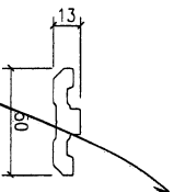
模號: X86504 名稱: 副框压块 合金狀態: 6063-T6 重量: 1.121 KG/M V.F.: -
