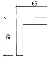
模號: X86516 名稱: 65x65x11.5mm鋁角 合金狀態: 6063-T6 重量: 3.693 KG/M V.F.: -
