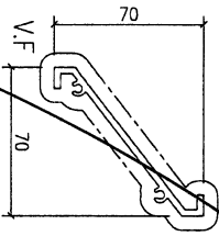
模號: X85958 名稱: 百叶片 合金狀態: 6063-T6 重量: 1.04 KG/M V.F.: 272.52mm
