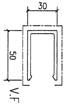
模號: X86511 名稱: 安全玻璃卡槽 合金狀態: 6063-T6 重量: 1.016 KG/M V.F.: 152.4
