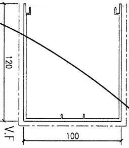
模號: X86495 名稱: 包鋼型材 合金狀態: 6063-T6 重量: 2.353 KG/M V.F.: 442.07mm
