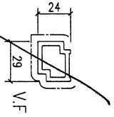
模號: X86513 名稱: 橫向墊高料 合金狀態: 6063-T6 重量: 0.764 KG/M V.F.: 71.93
