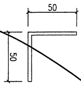
模號: JM1001 名稱: 50x50x3mm鋁角 合金狀態: 6063-T6 重量: 0.852 KG/M V.F.: -
