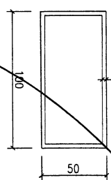
模號: JMF00032R30 名稱: 100x50x3mm鋁通 合金狀態: 6063-T6 重量: 2.528 KG/M V.F.: -
