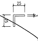
模號: JM1015 名稱: 25x25x3mm鋁角 合金狀態: 6063-T6 重量: 0.413 KG/M V.F.: -
