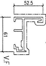
模號: X86505 名稱: 开窗竖向内框 合金狀態: 6063-T6 重量: 1.442 KG/M V.F.: 208.97mm
