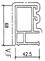
模號: X86503 名稱: 开窗橫向外框 合金狀態: 6063-T6 重量: 2.071 KG/M V.F.: 191.08mm
