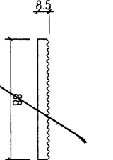
模號: X86514 名稱: 碼件墊片 合金狀態: 6061-T6 重量: 1.789 KG/M V.F.: -
