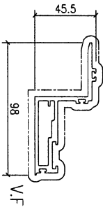
模號: X86506 名稱: 开窗竖向窗扇 合金狀態: 6063-T6 重量: 1.722 KG/M V.F.: 332.86mm
