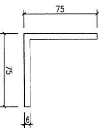
模號: JM1079 名稱: 75x75x6mm铝角 合金狀態: 6063-T6 重量: 2.539 KG/M V.F.: -
