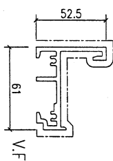
模號: X86509 名稱: 开窗向内框 合金狀態: 6063-T6 重量: 1.503 KG/M V.F.: 225.21mm
