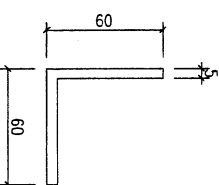
模號: X86514 名稱: 码件垫片 合金狀態: 6061-T6 重量: 1.789 KG/M V.F.: -
