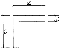
模號: X86516 名稱: 65x65x11.5mm铝角 合金狀態: 6063-T6 重量: 3.693 KG/M V.F.: -
