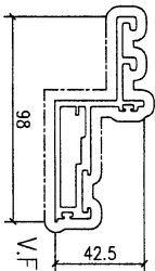
模號: X86507 名稱: 开窗横向窗扇 合金狀態: 6063-T6 重量: 1.849 KG/M V.F.: 353.78mm
