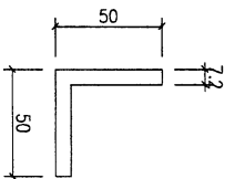
模號: X86515 名稱: 50x50x7.2mm铝角 合金狀態: 6063-T6 重量: 1.811 KG/M V.F.: -
