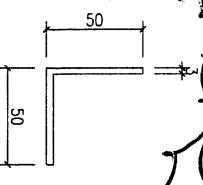
模號: JM1001 名稱: 50x50x3mm铝角 合金狀態: 6063-T6 重量: 0.852 KG/M V.F.: -
