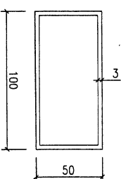
模號: JMF0032B30 名稱: 100x50x3mm铝通 合金狀態: 6063-T6 重量: 2.528 KG/M V.F.: -
