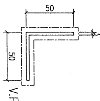
模號: JM1001 名稱: 50x50x3mm铝角 合金狀態: 6063-T6 重量: 0.852 KG/M V.F.: 200
