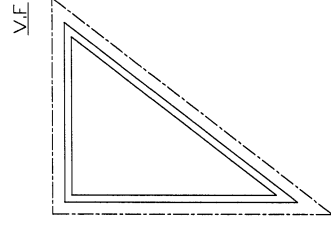
模號: X86545 名稱: 裝飾條 合金狀態: 6063-T6 重量: 2.257 KG/M V.F.: 293 mm
