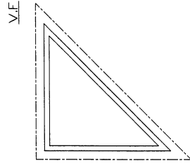
模號: X86544 名稱: 裝飾條 合金狀態: 6063-T6 重量: 1.94 KG/M V.F.: 253 mm
