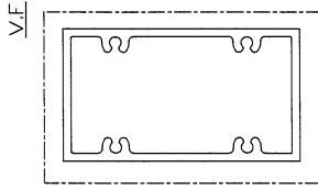
模號: X86540 名稱: 裝飾條 合金狀態: 6063-T6 重量: 2.594 KG/M V.F.: 280 mm
