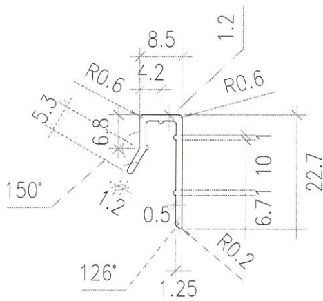
SCALE 1:1
