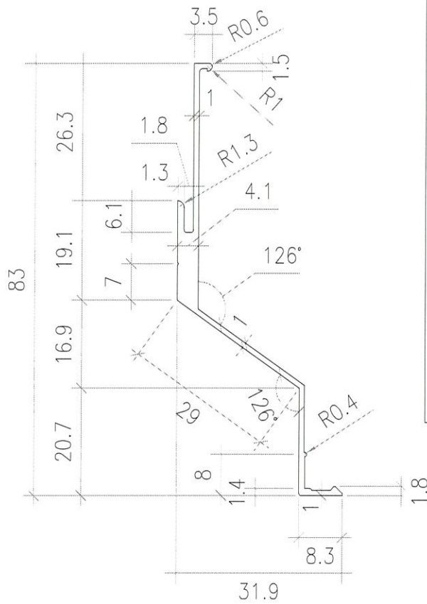
SCALE 1:1
