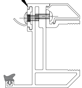
窗玉扣碼墊巴 安裝示意圖 (ALB-04)
