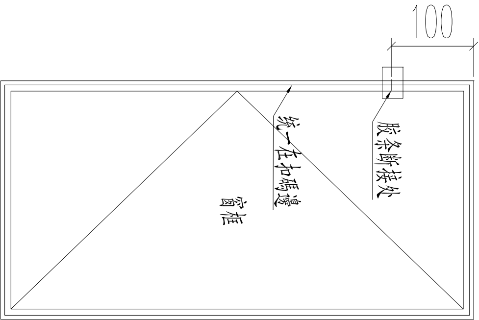
框上胶条接口示意图
