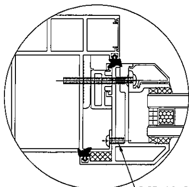
M5x10圓頭機絲
