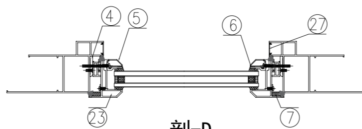
剖-D
