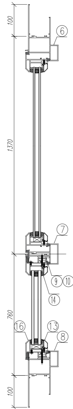
剖-A
