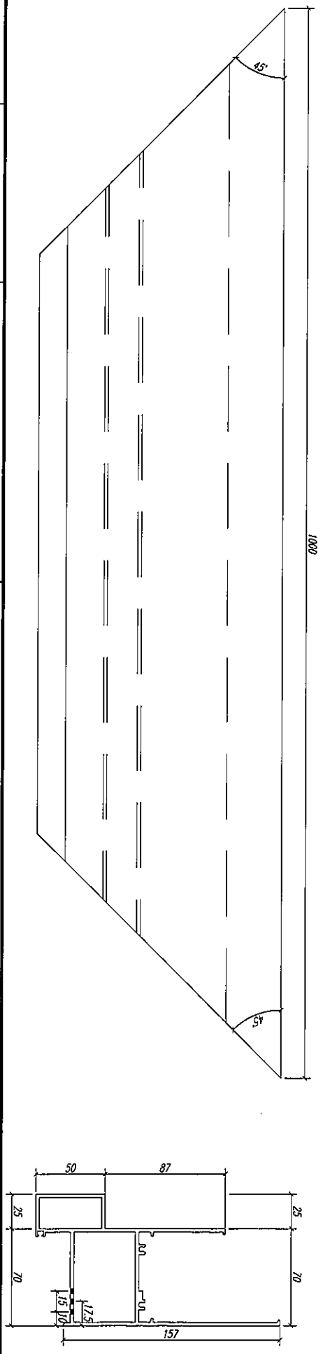
右视图2
