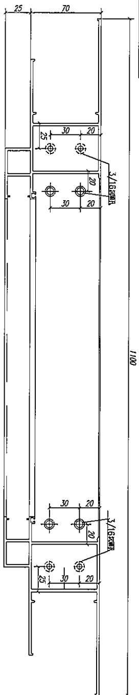
右视图1
