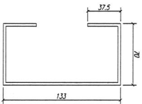
鋁折件3
