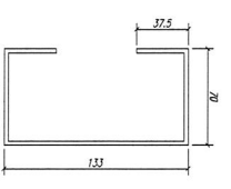
鋁折件3
