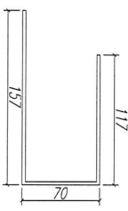
鋁折件12
