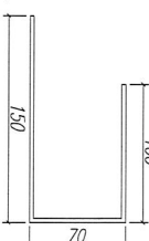
鋁折件4
