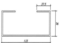
鋁折件10
