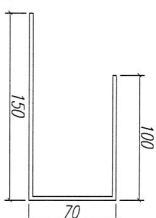
鋁折件6
