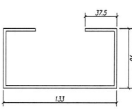
鋁折件3
