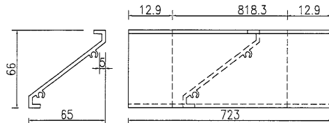
④號百葉加工圖
