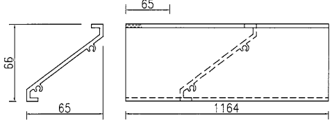
③號百葉加工圖
