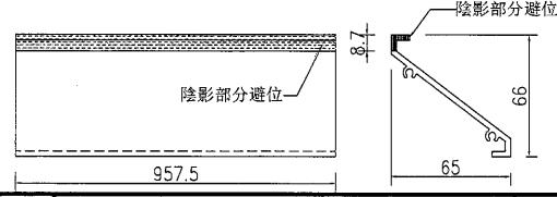
號百葉加工圖③
