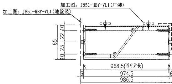
①號百葉加工圖
