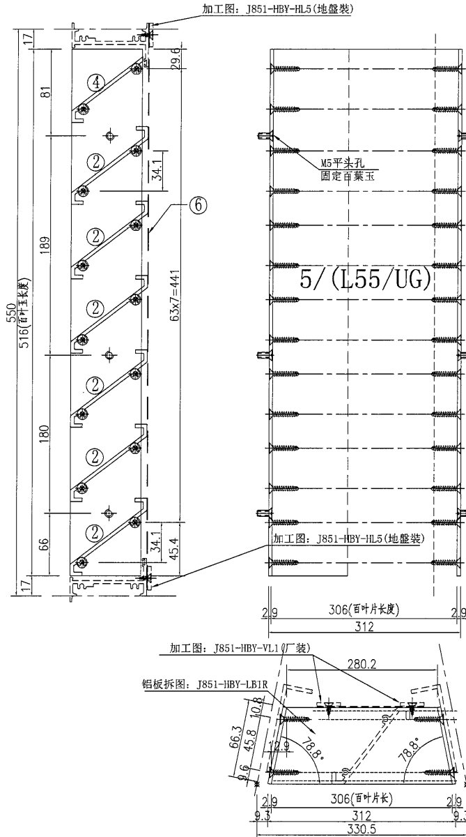
②號百葉加工圖
