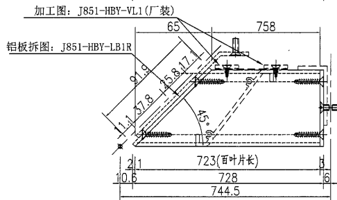
②號百葉加工圖
