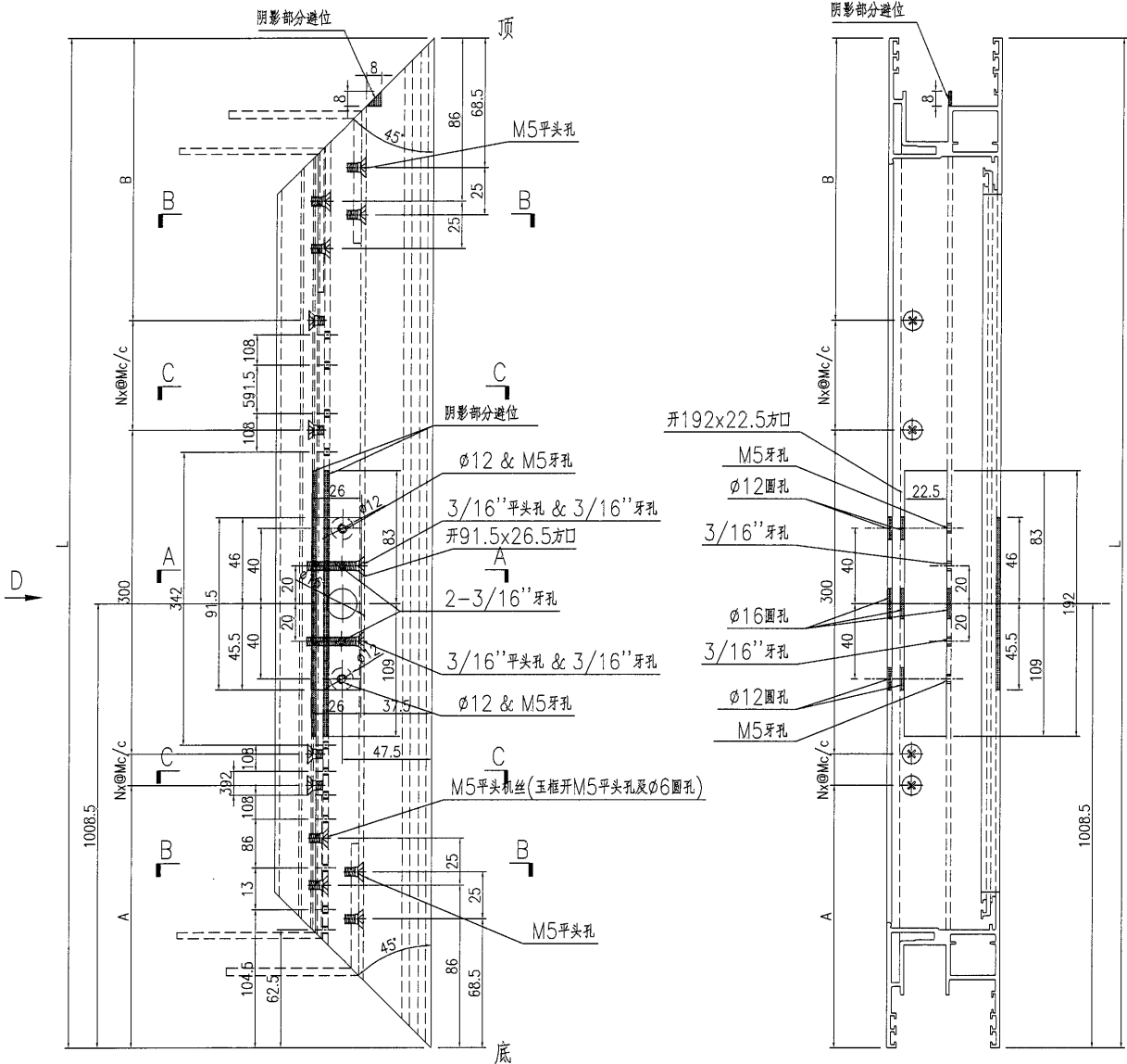
D-D视图
