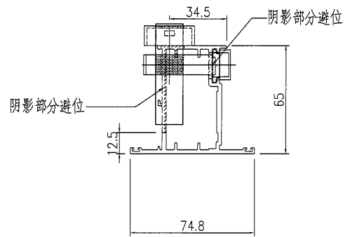
锁芯安装示意图 (锁芯配孔需以实物为准)
