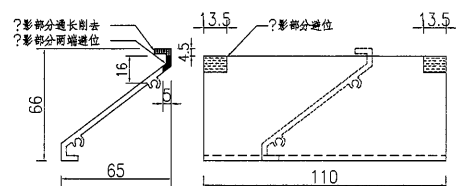
②?百?加工?
