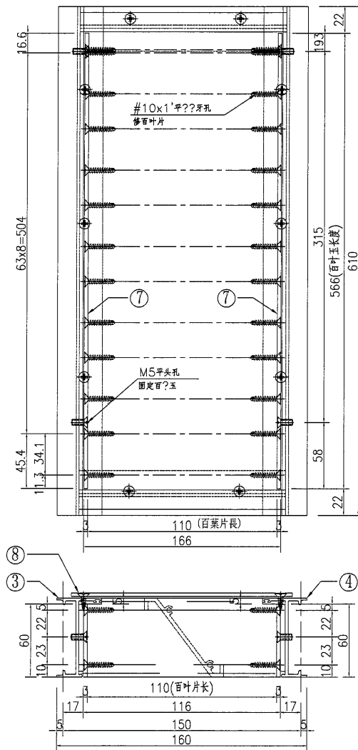
②?百?加工?
