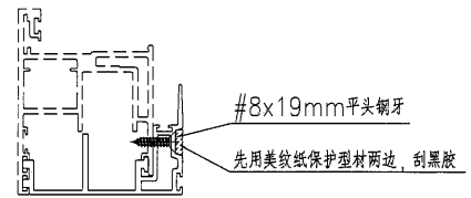
工厂型材组装示意图
