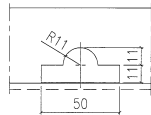
排水孔尺寸
