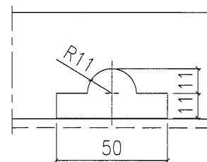
排水孔尺寸
