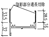
切料圖
