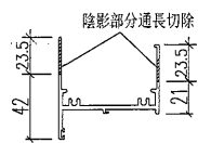
切料圖
