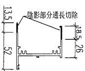
切料圖
