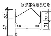
切料圖
