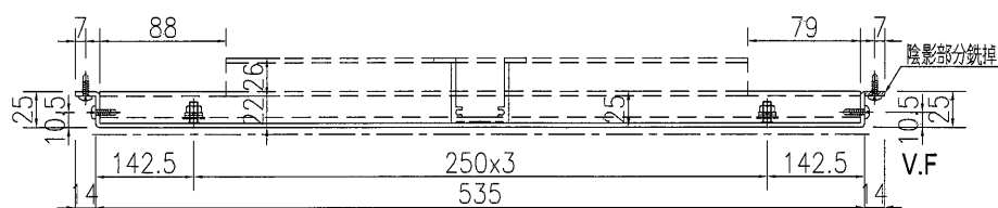
SECTION A-A
