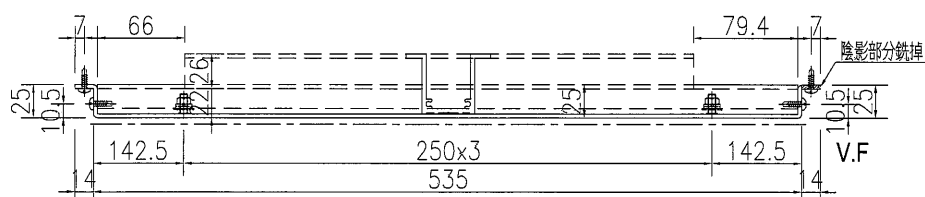
SECTION A-A
