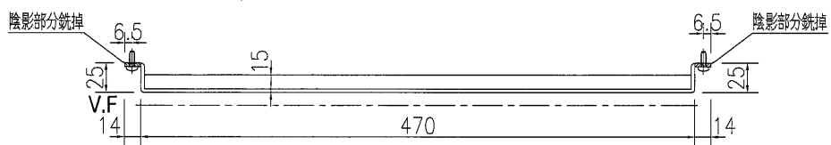
SECTION A-A
