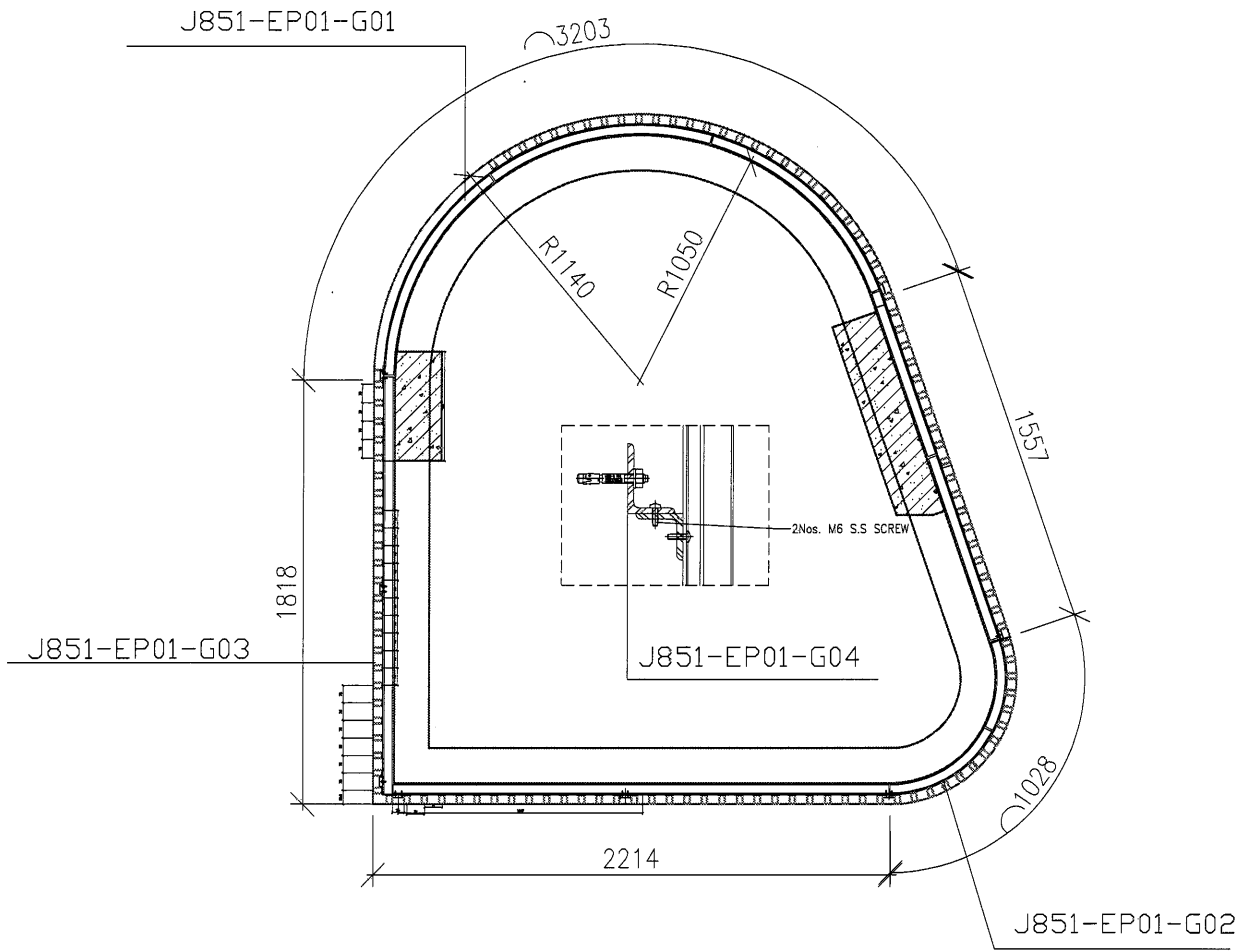
格栅平面圖
