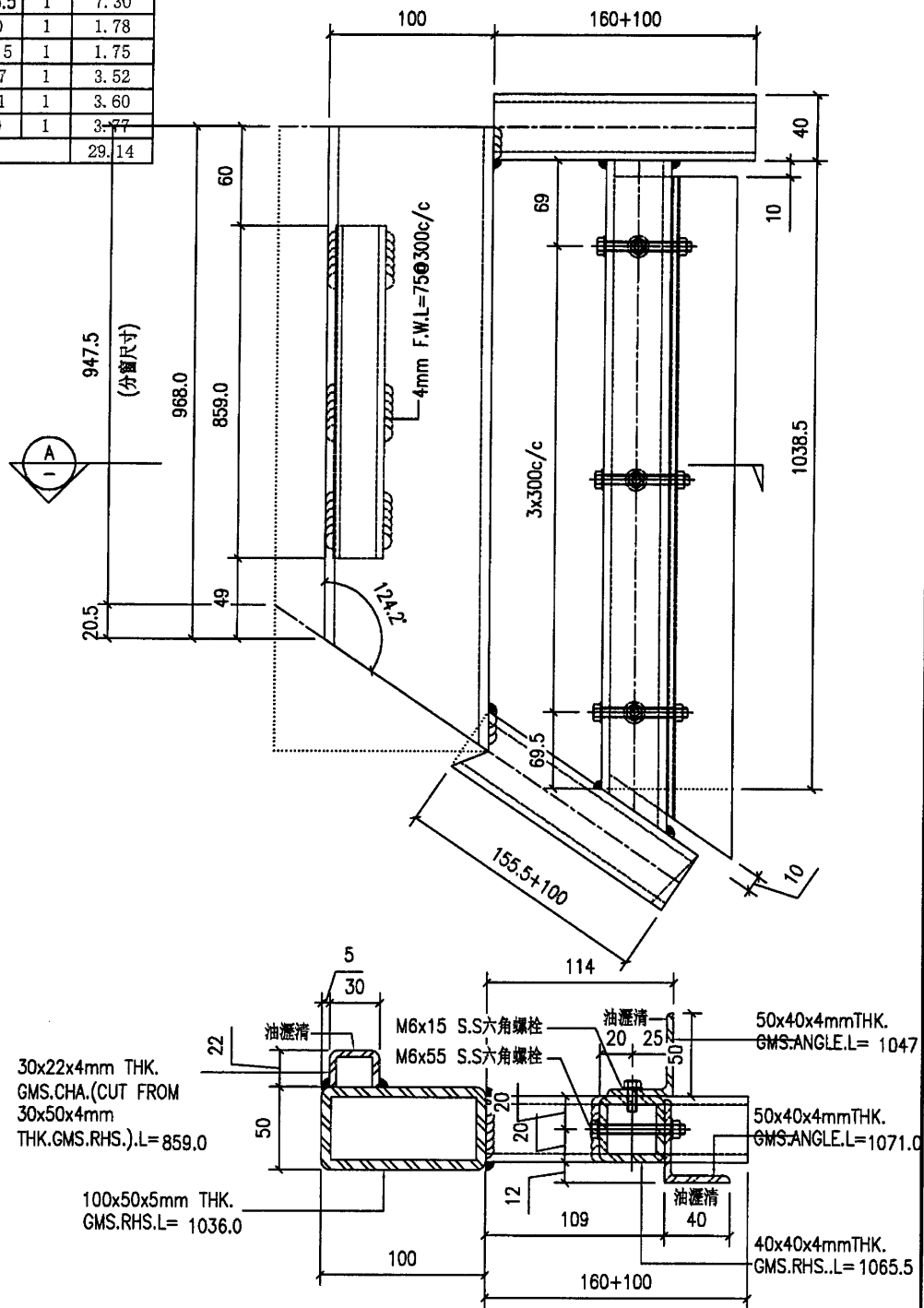
SECTION A-A
