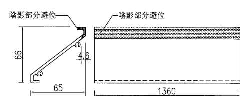
②號百葉加工圖
