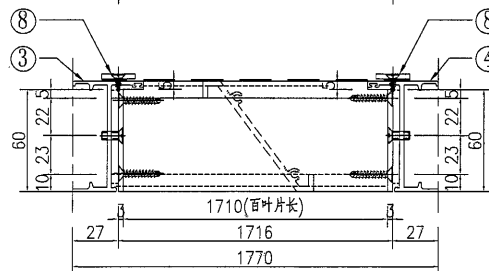
②號百葉加工圖
