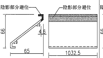
③號百葉加工圖
