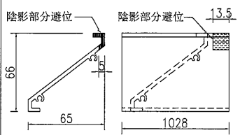
②號百葉加工圖
