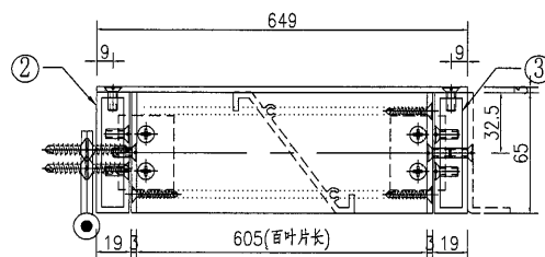
①號百葉加工圖
