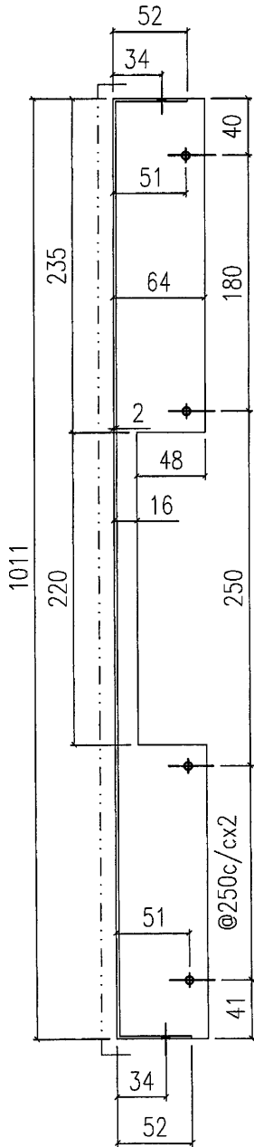
SECTION A-A
