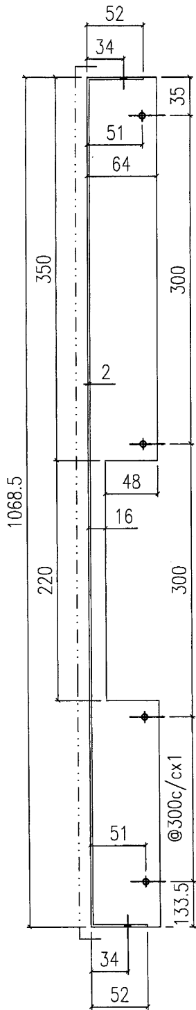
SECTION A-A
