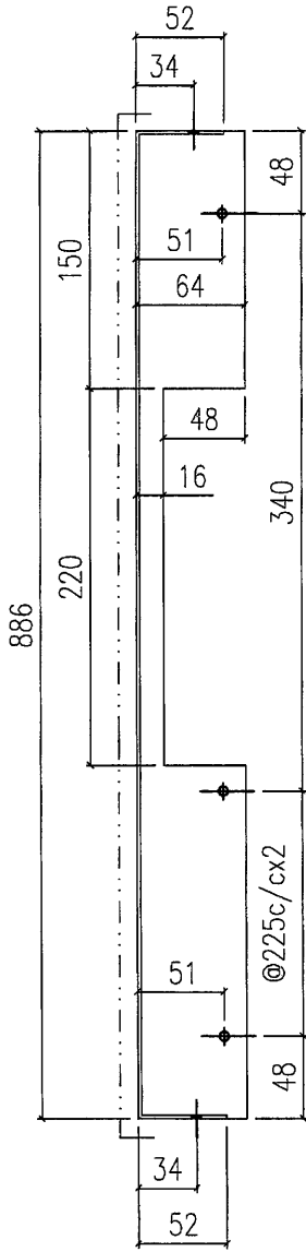
SECTION A-A
