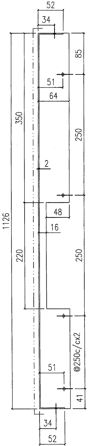
SECTION A-A
