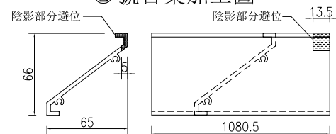
④號百葉加工圖
