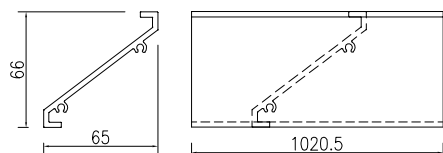
①號百葉加工圖
