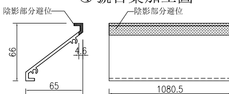
④號百葉加工圖
