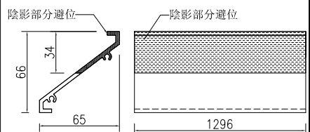
③號百葉加工圖
