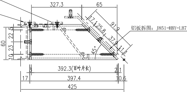
②號百葉加工圖
