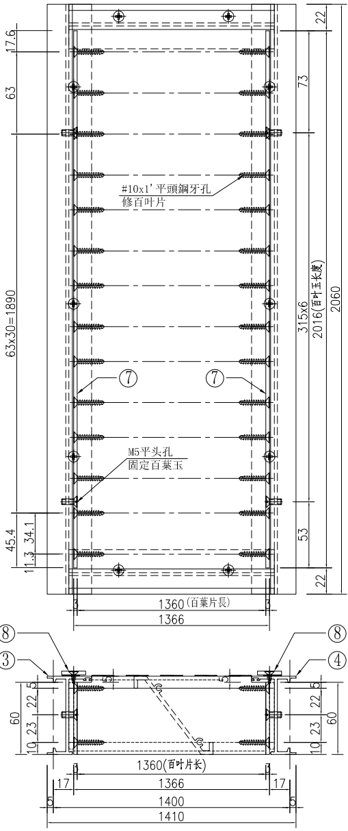
②號百葉加工圖
