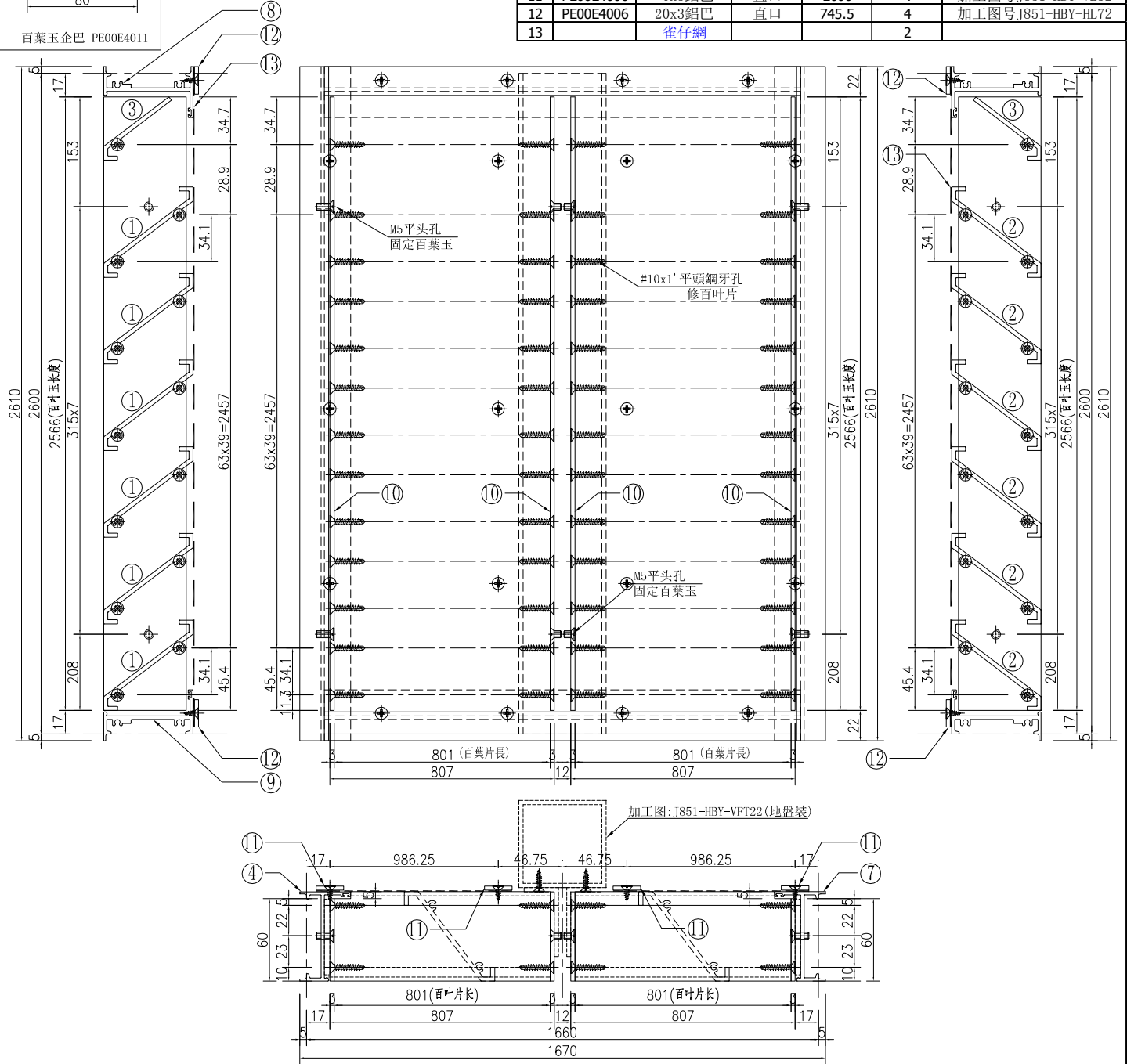
①號百葉加工圖
