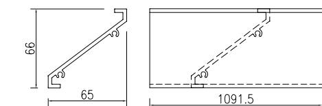
③號百葉加工圖
