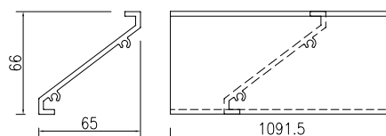
④號百葉加工圖
