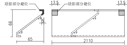
①號百葉加工圖
