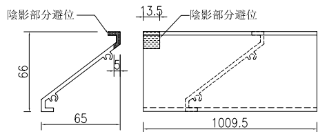
③號百葉加工圖
