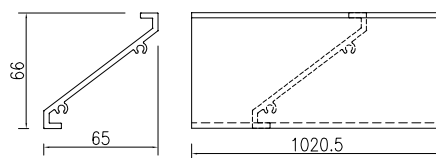
④號百葉加工圖
