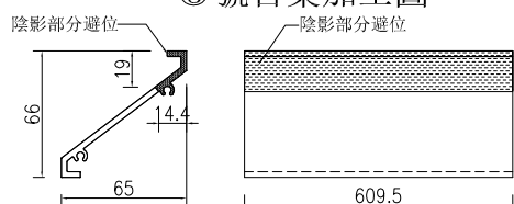
③號百葉加工圖
