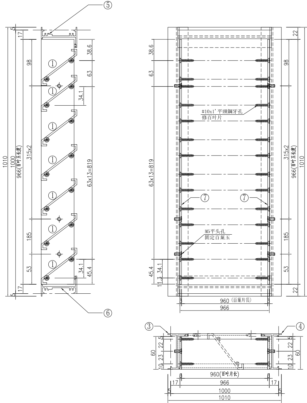
①號百葉加工圖
