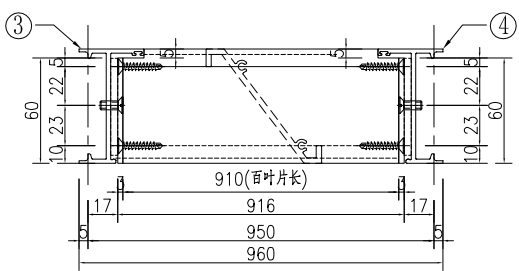
②號百葉加工圖
