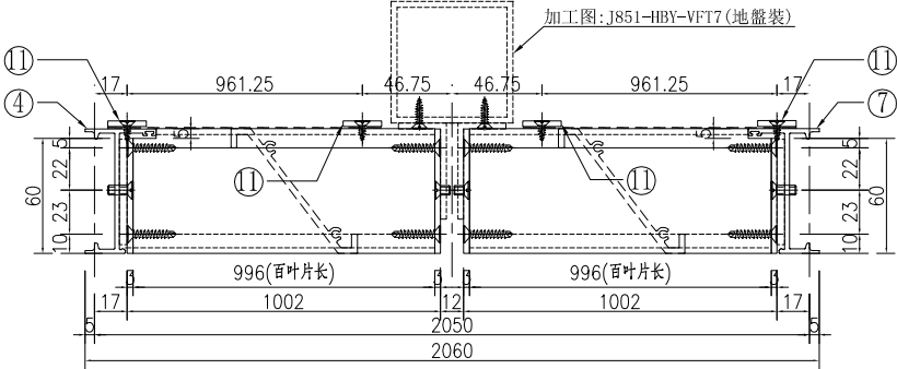
②號百葉加工圖
