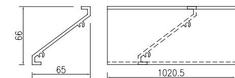
③號百葉加工圖
