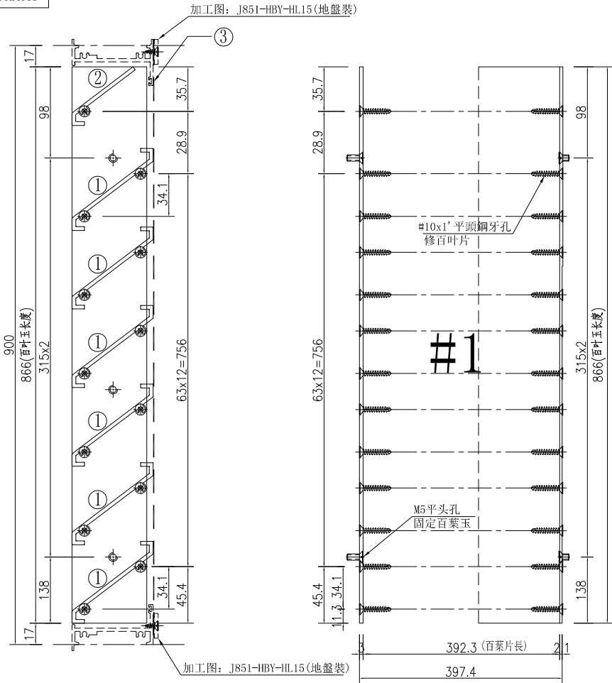
加工圖: J851-HBY-VL33 (廠裝)
