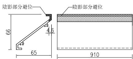
②號百葉加工圖
