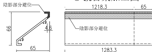
④號百葉加工圖
