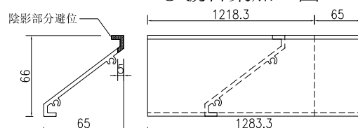
④號百葉加工圖
