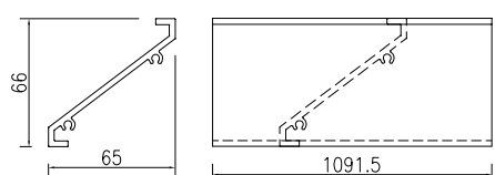
①號百葉加工圖
