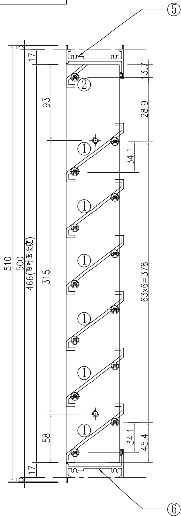
百葉玉企巴 PE00E4011
