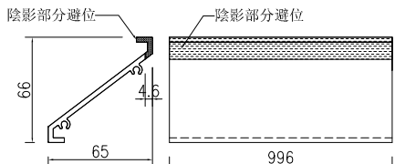
③號百葉加工圖
