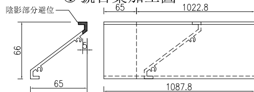
③號百葉加工圖
