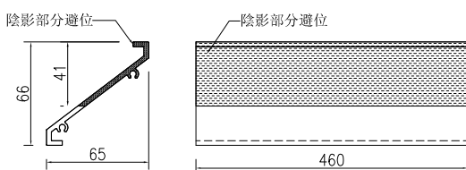
②號百葉加工圖
