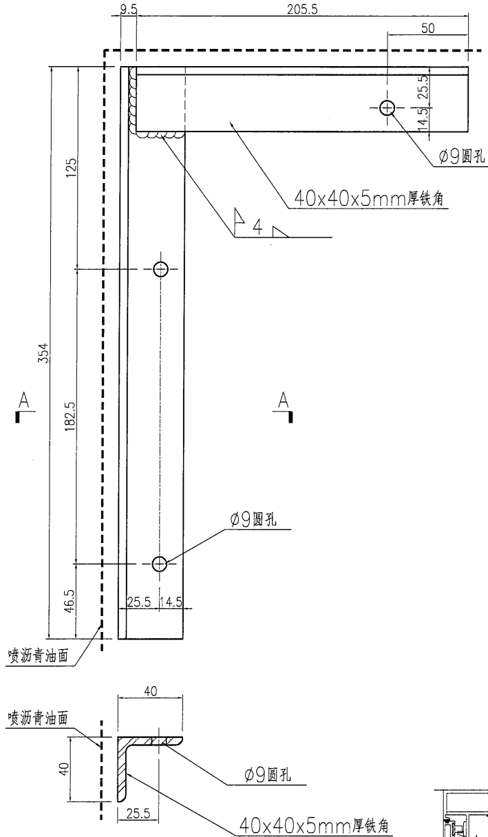
SECTION A-A
