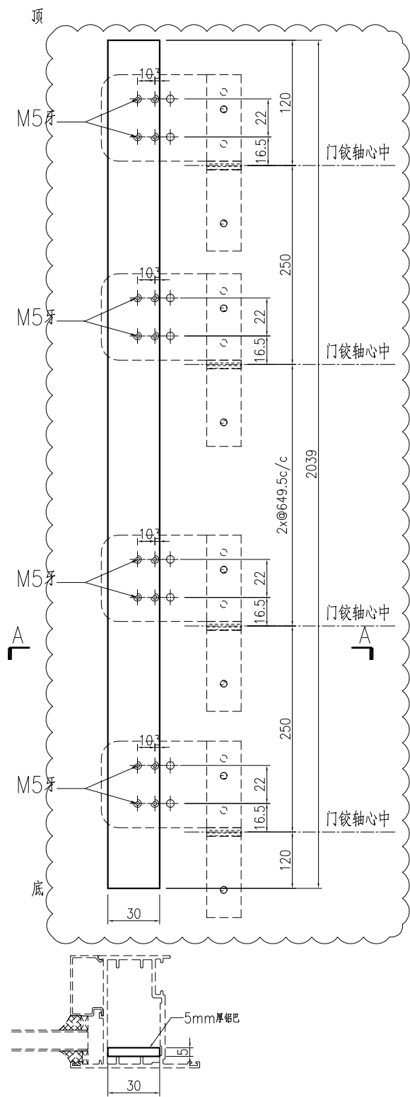
SECTION A-A
