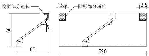
①號百葉加工圖
