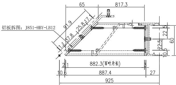
①號百葉加工圖
