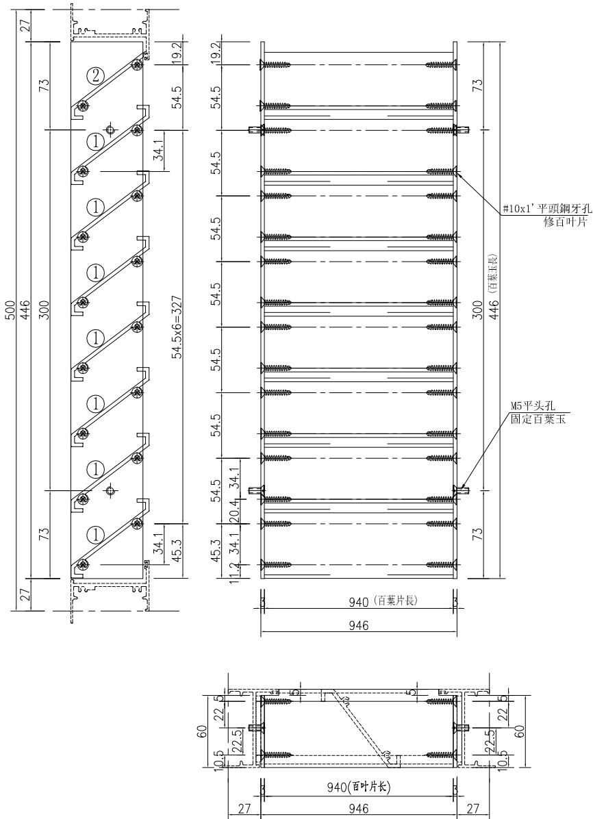
①號百葉加工圖
