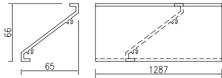
③號百葉加工圖
