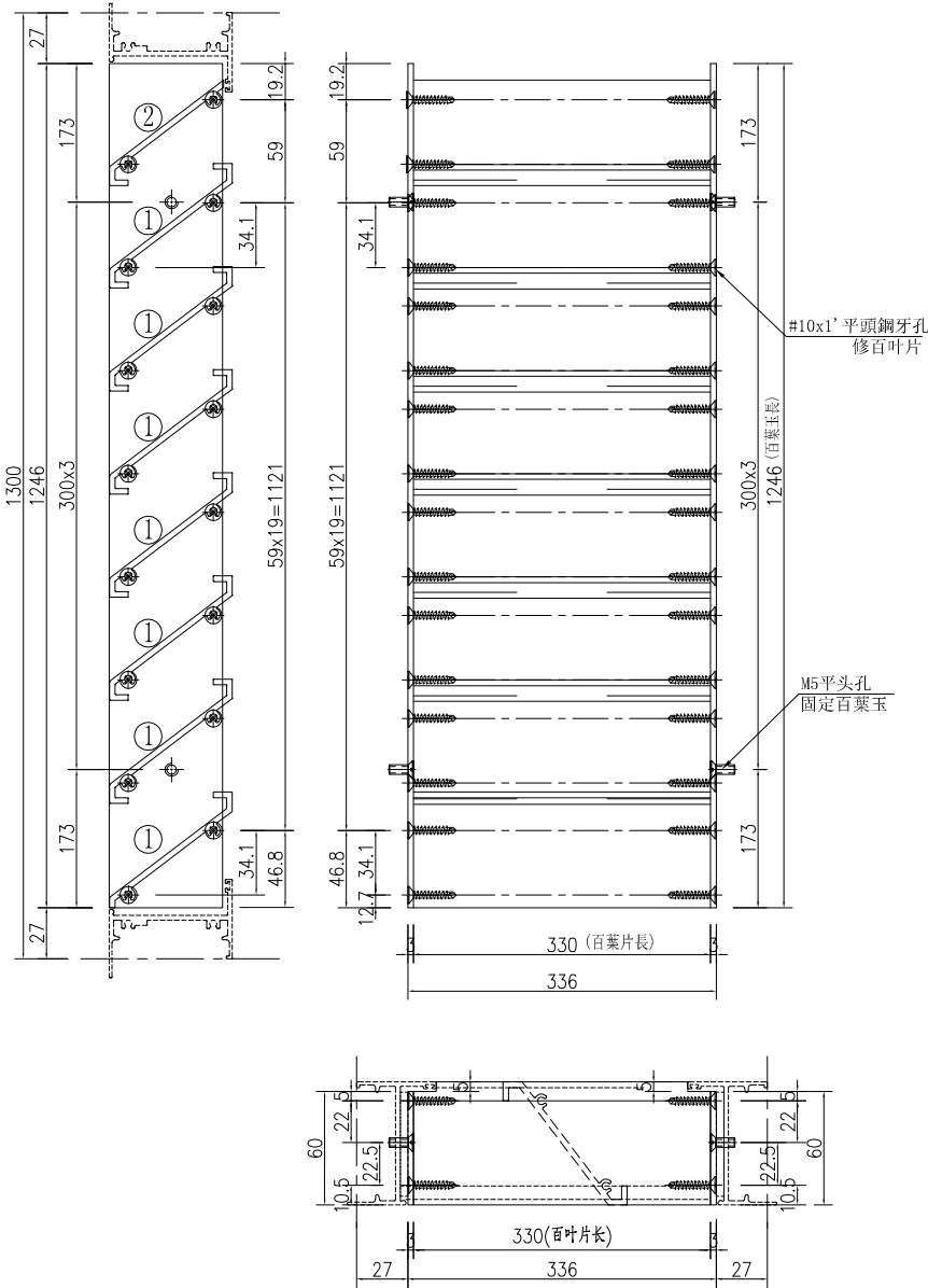
①號百葉加工圖
