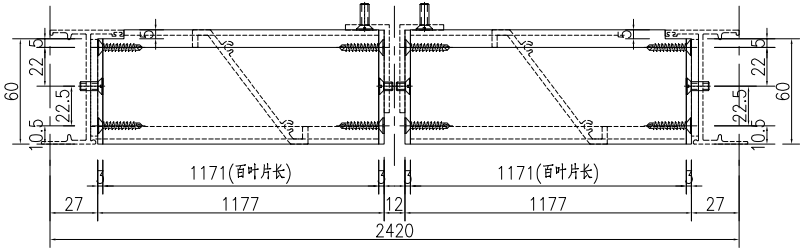
②號百葉加工圖
