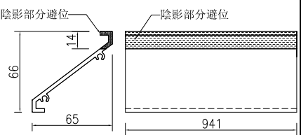
③號百葉加工圖
