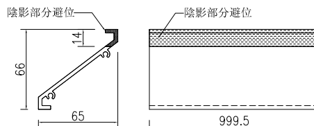
④號百葉加工圖
