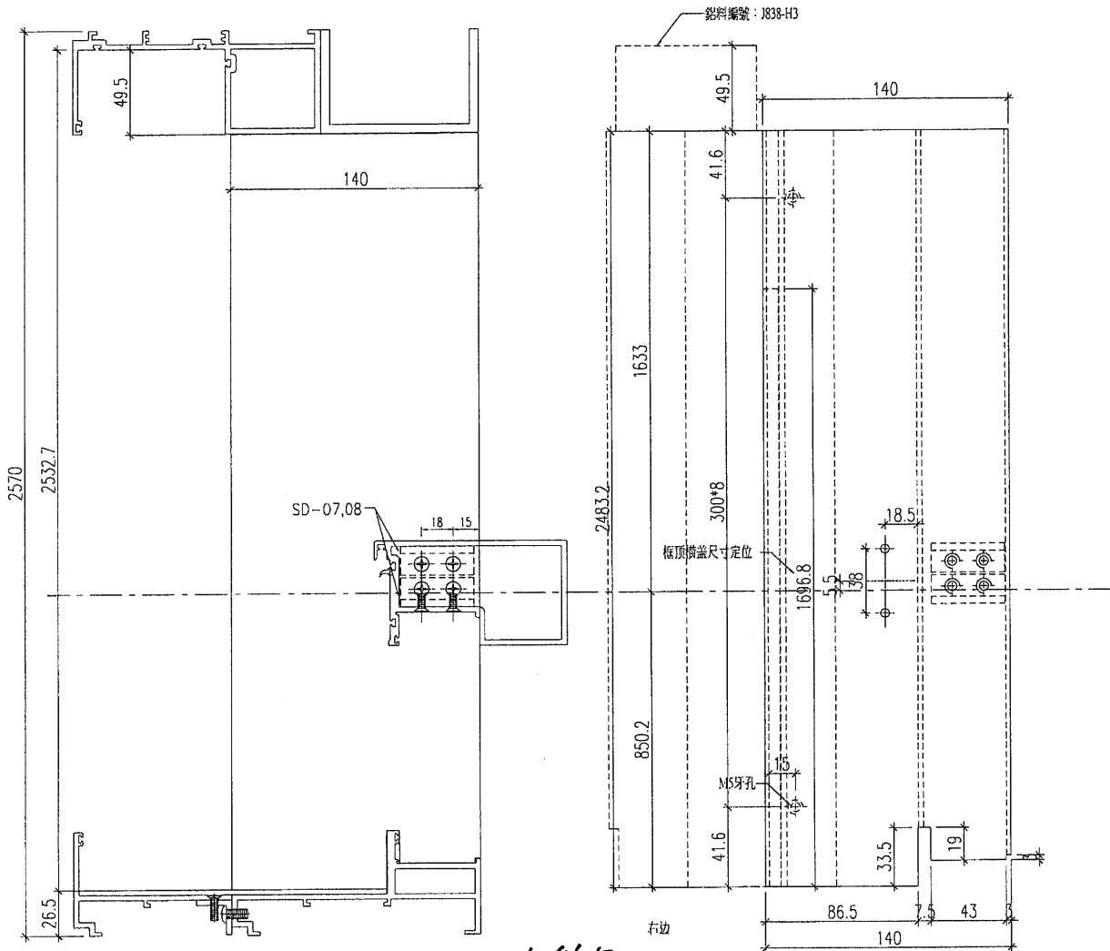
組裝示意圖
